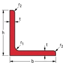
تصویر 1: نمای کلی نبشی بال مساوی
