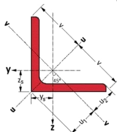
تصویر 1: نمای کلی نبشی بال مساوی
