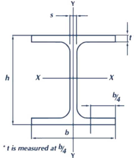
تصویر 2: نمای کلی مقاطع فولادی H 0
