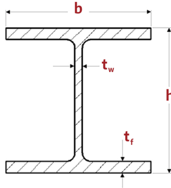
تصویر 1: نمای کلی تیرآهن بال پهن
