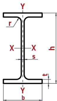
تصویر 1: نمای کلی تیرآهن با لبه موازی (IPE)
