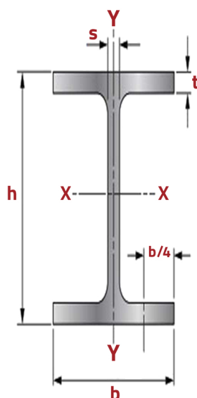
تصویر 2: نمای کلی تیرآهن با لبه موازی (IPE)
